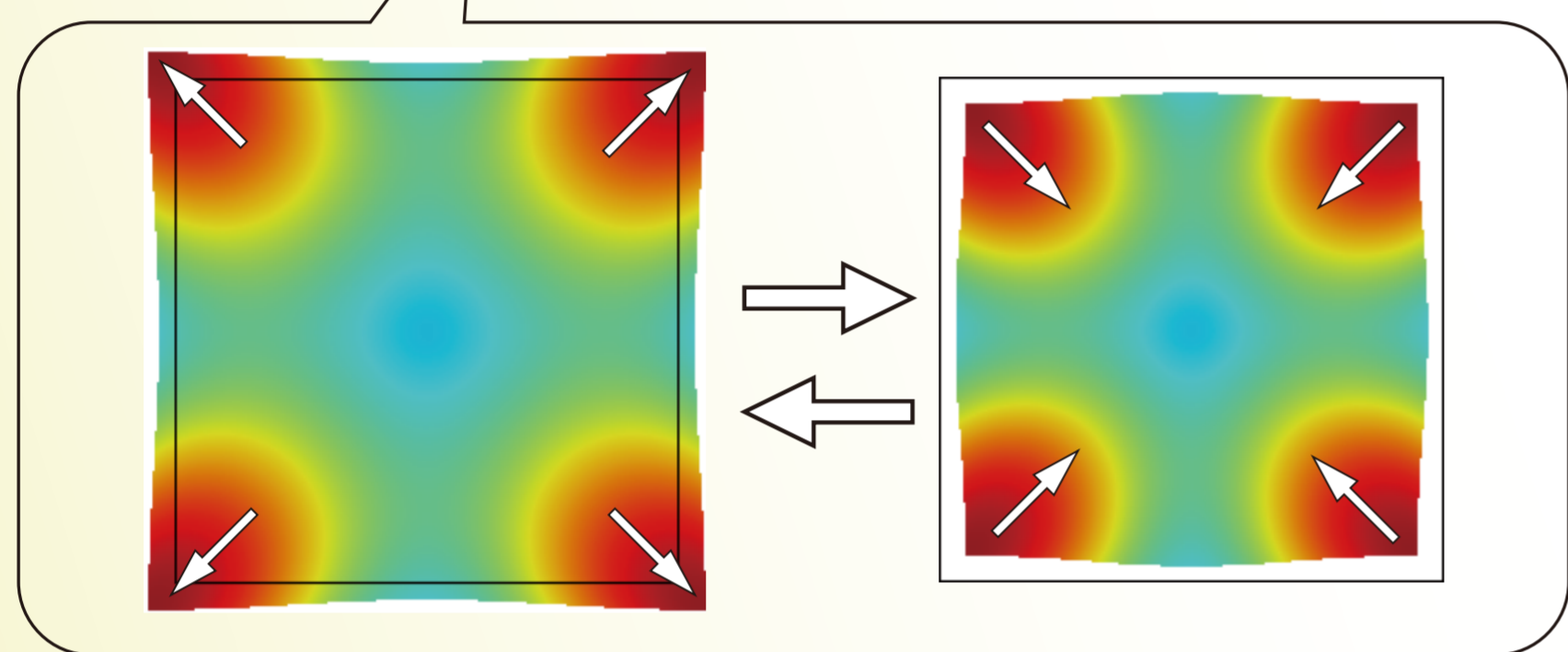
正方形の面内呼吸モード
