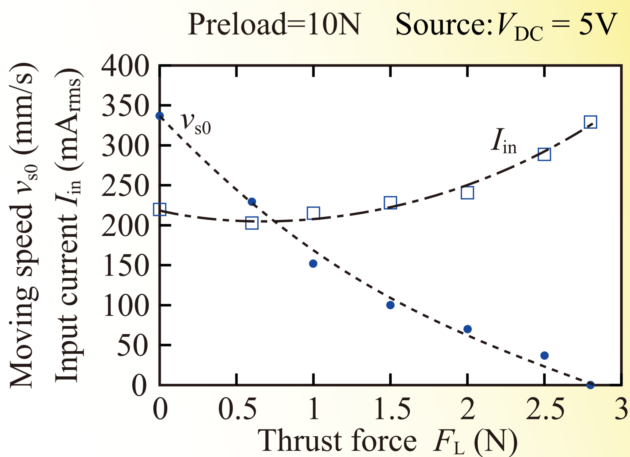
リニア型モータの特性例
