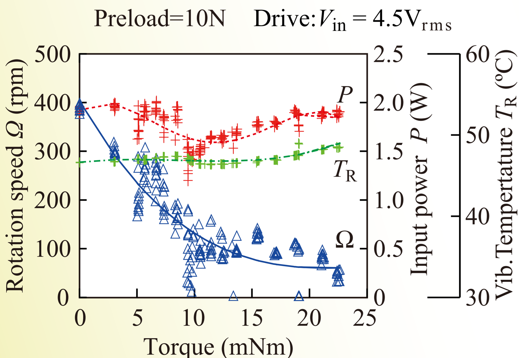
回転型モータの特性例(連続回転)
