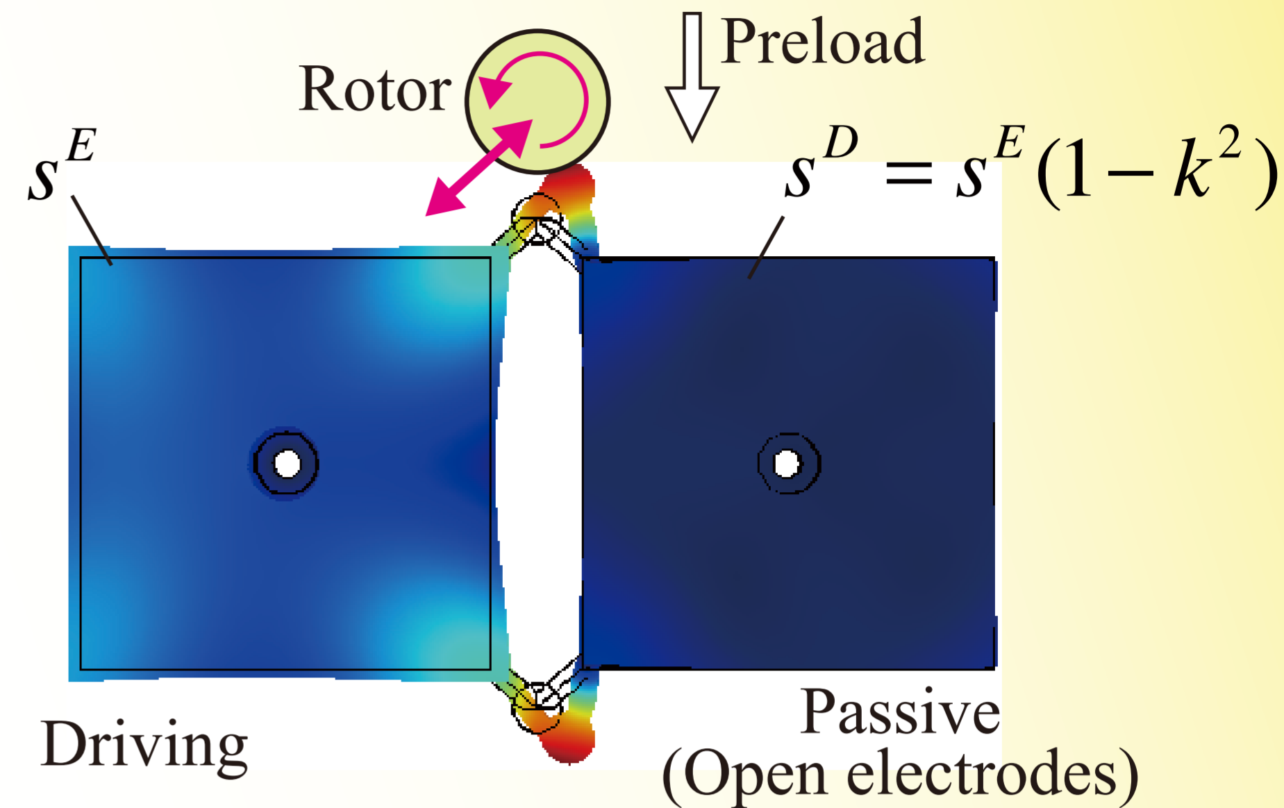
左側正方形のみ駆動→左回転
