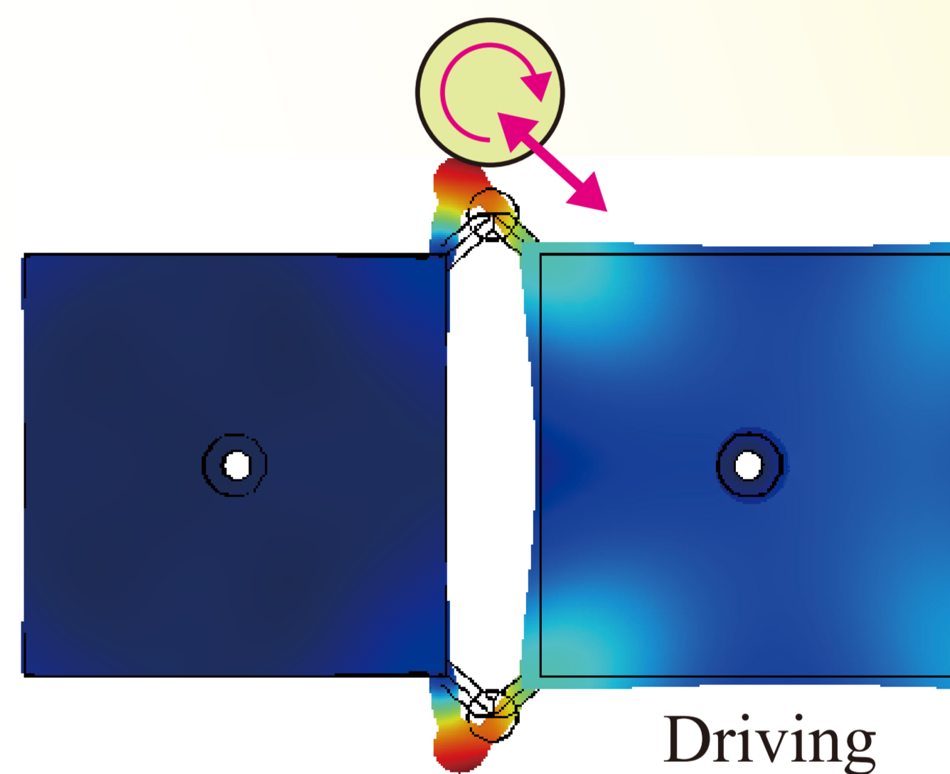
右側正方形のみ駆動→右回転
