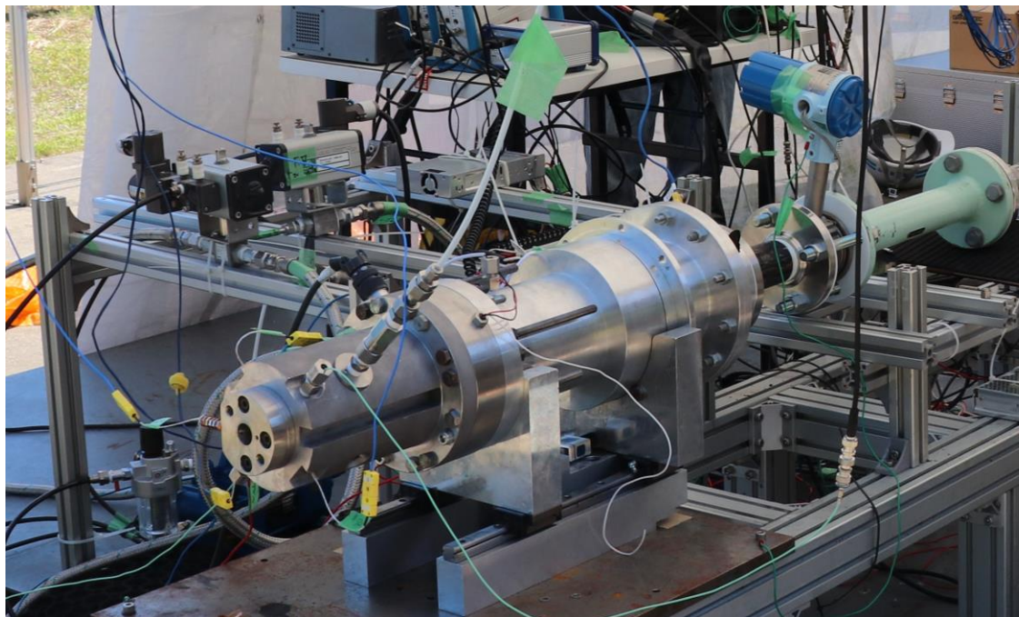
衝突噴流エンジン
