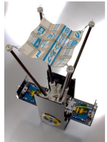
超小型衛星「ひろがり」（展開時）
