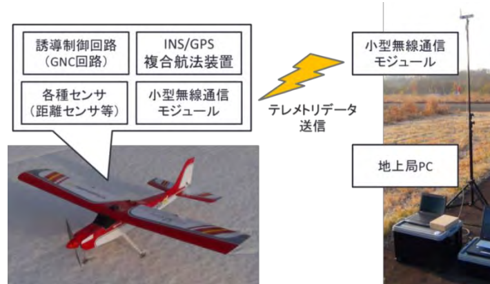
図 4 実験機器構成
