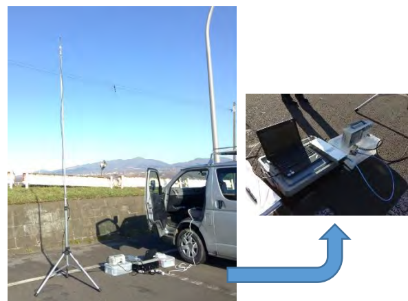
図8 本格版受信系設置状況(8.6 km)
