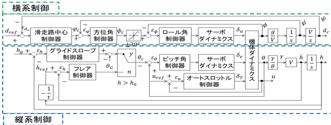
図3 着陸制御系
