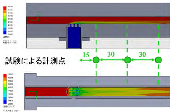
図 4-1 整列配置の冷却ガス分布
