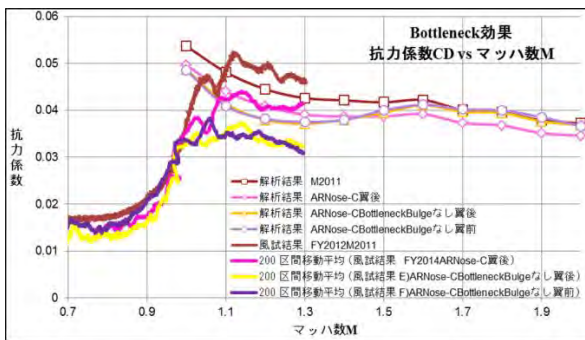
図 10 風洞試験および解析における bottleneck の効果
