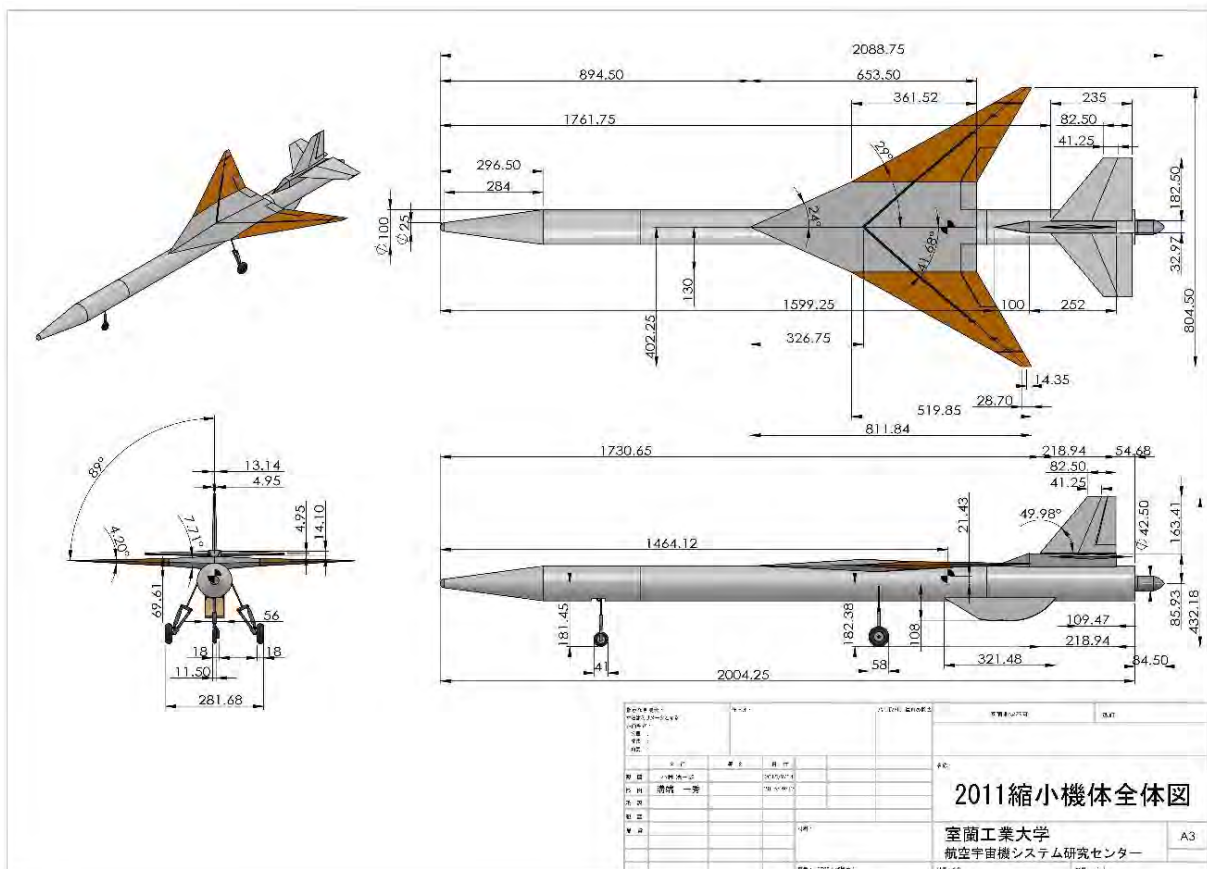
図 1 第二世代オオワシ 1/3 スケール縮小機体の設計図面
