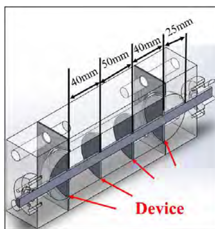
図 2-3 試験等タンクおよび内部デバイス
