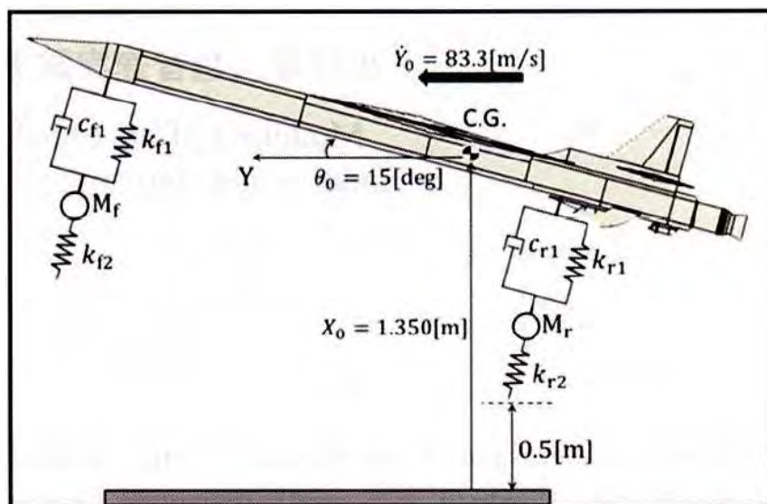
図1 脚柱1本構造案2次元モデル
