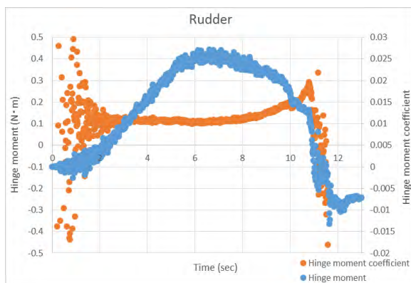
(c) ラダー
